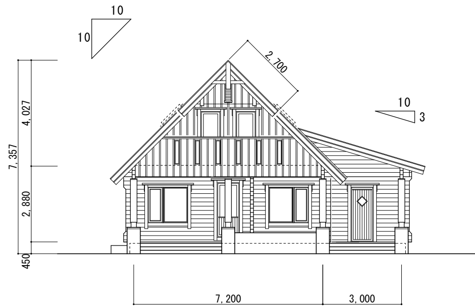
立面图 S=1/100
