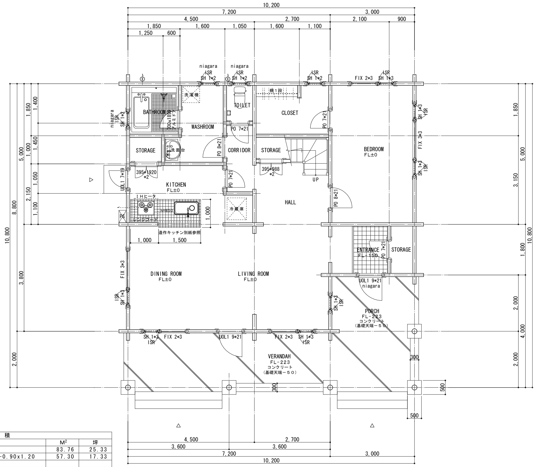
1階平面図 S=1/50
