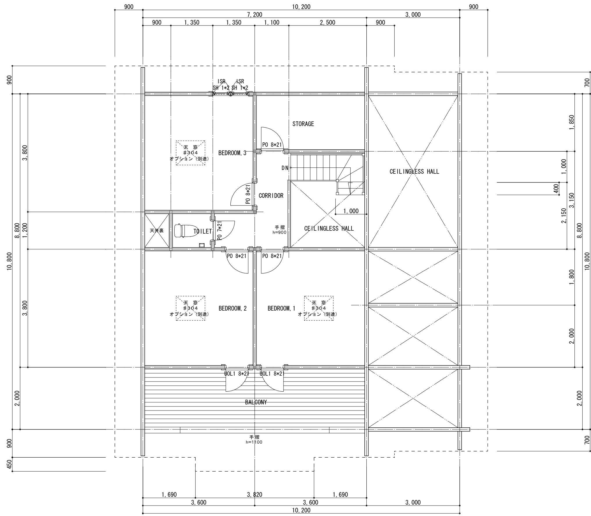
2階平面図 S=1/50
