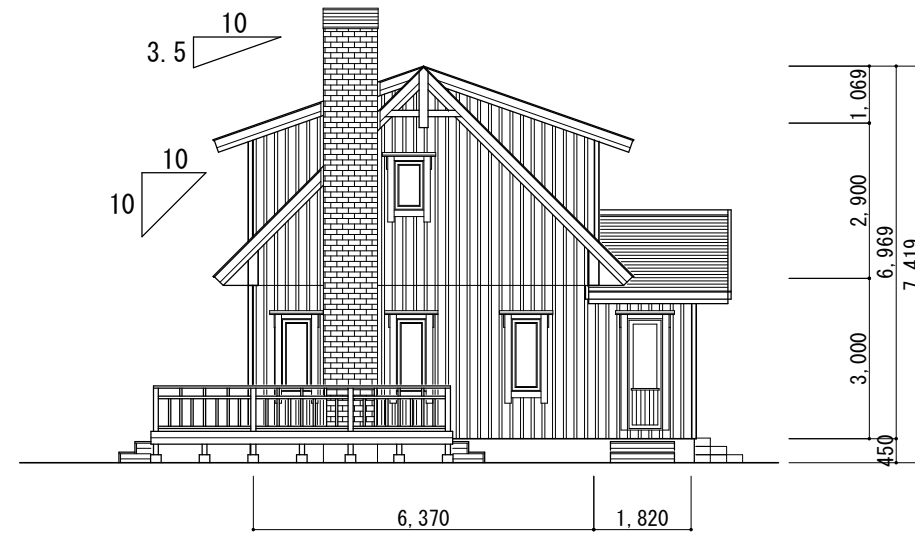
東側立面图 S=1/100
