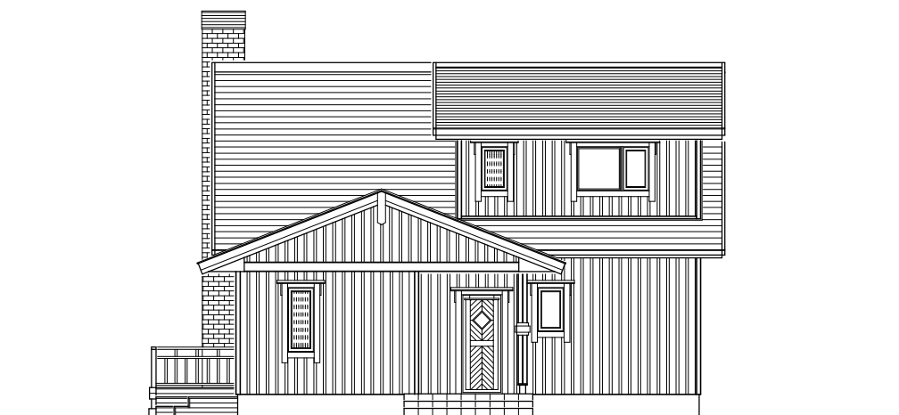
北側立面图 S=1/100
