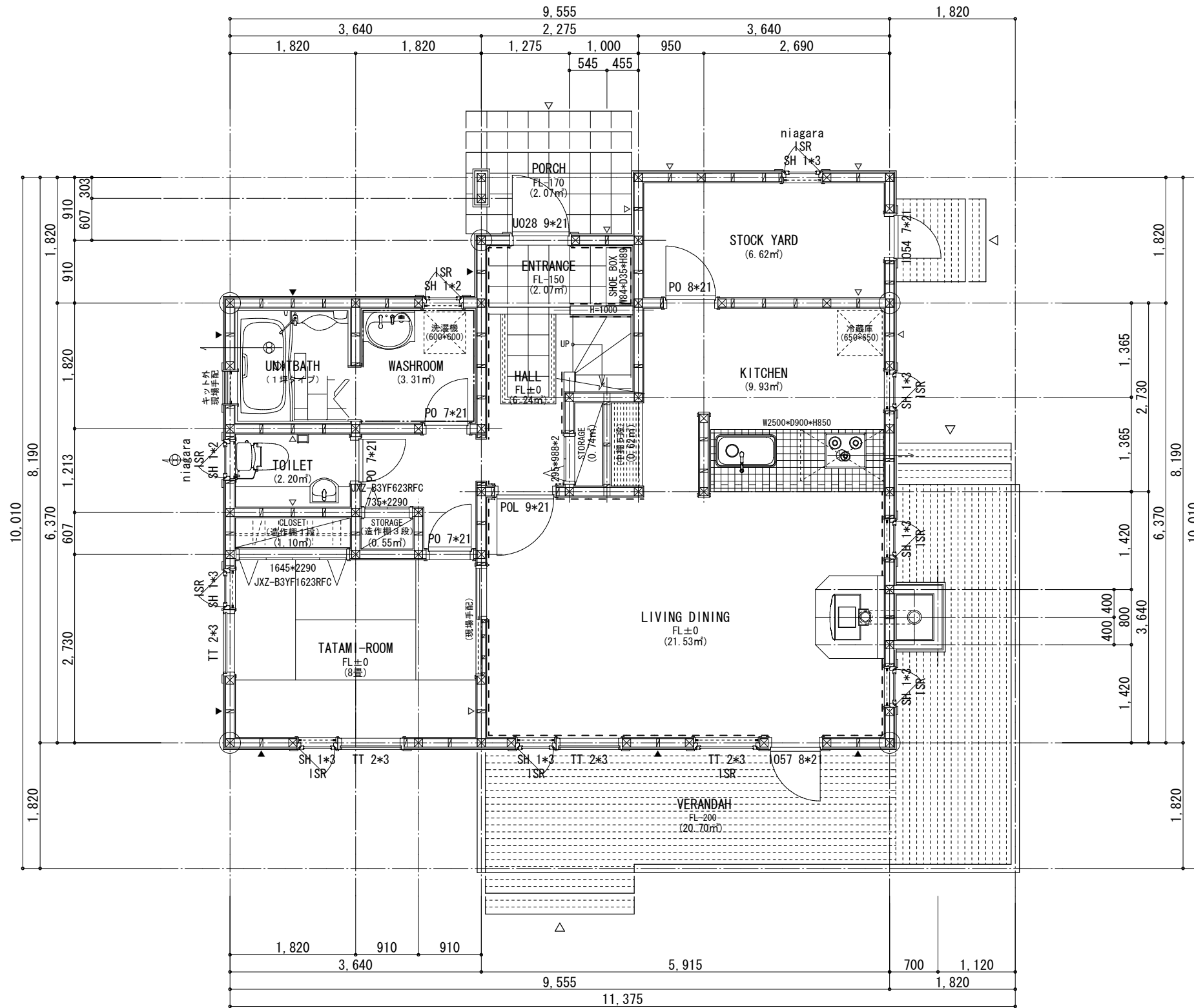
1階平面図 S=1/50
