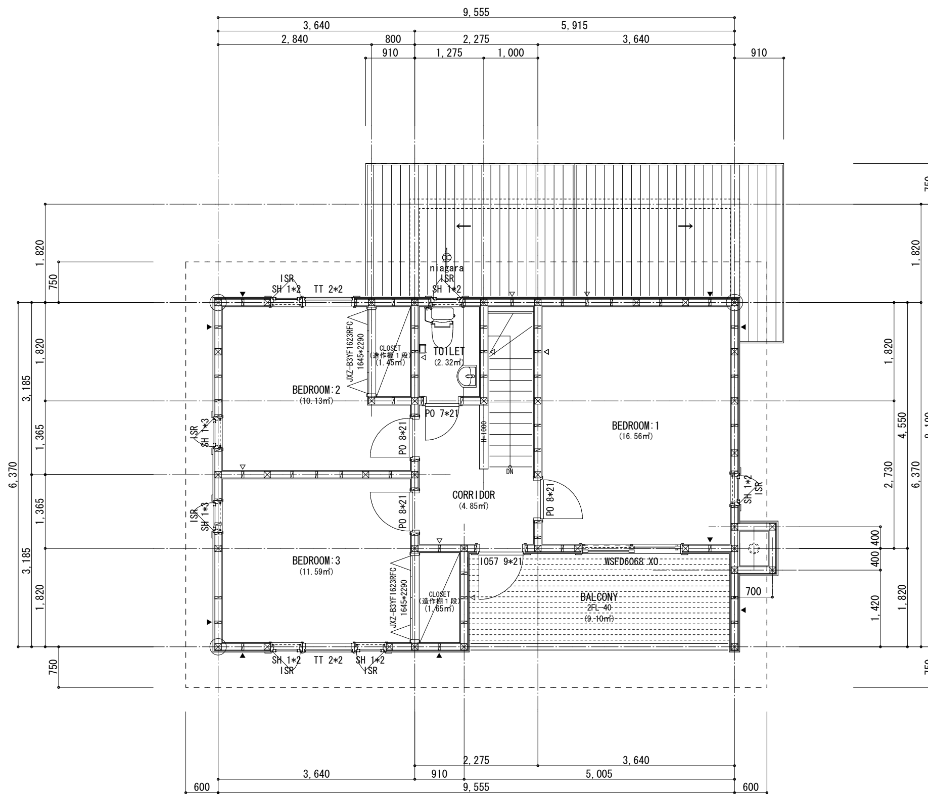
2階平面図 S=1/50
