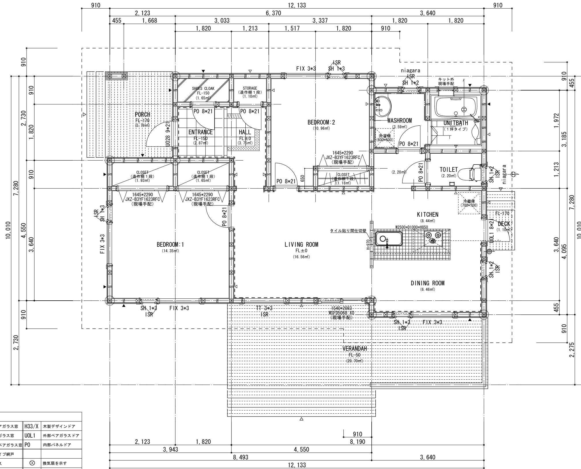
平面図 S=1/50
