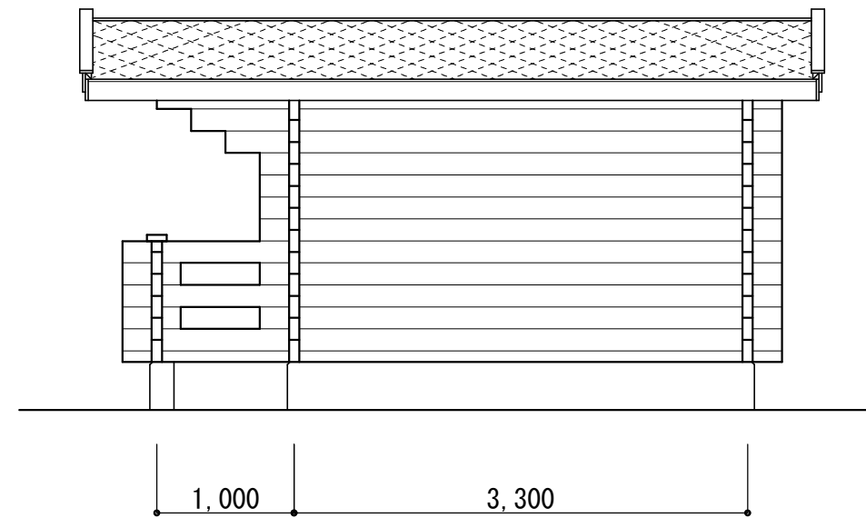
立面图 S=1/50
