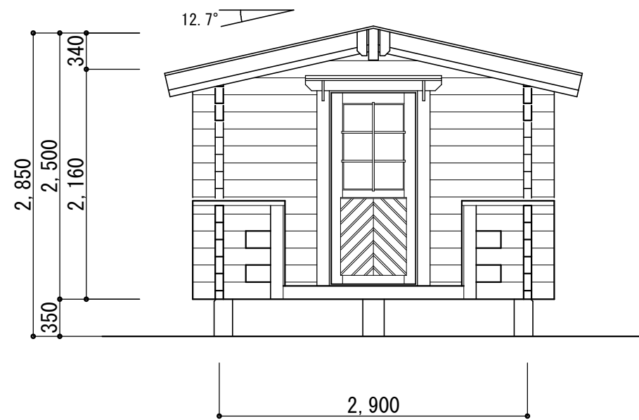
立面图 S=1/50
