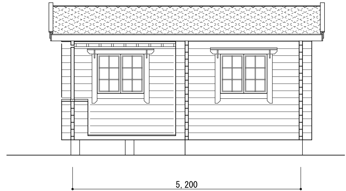
立面图 S=1/50
