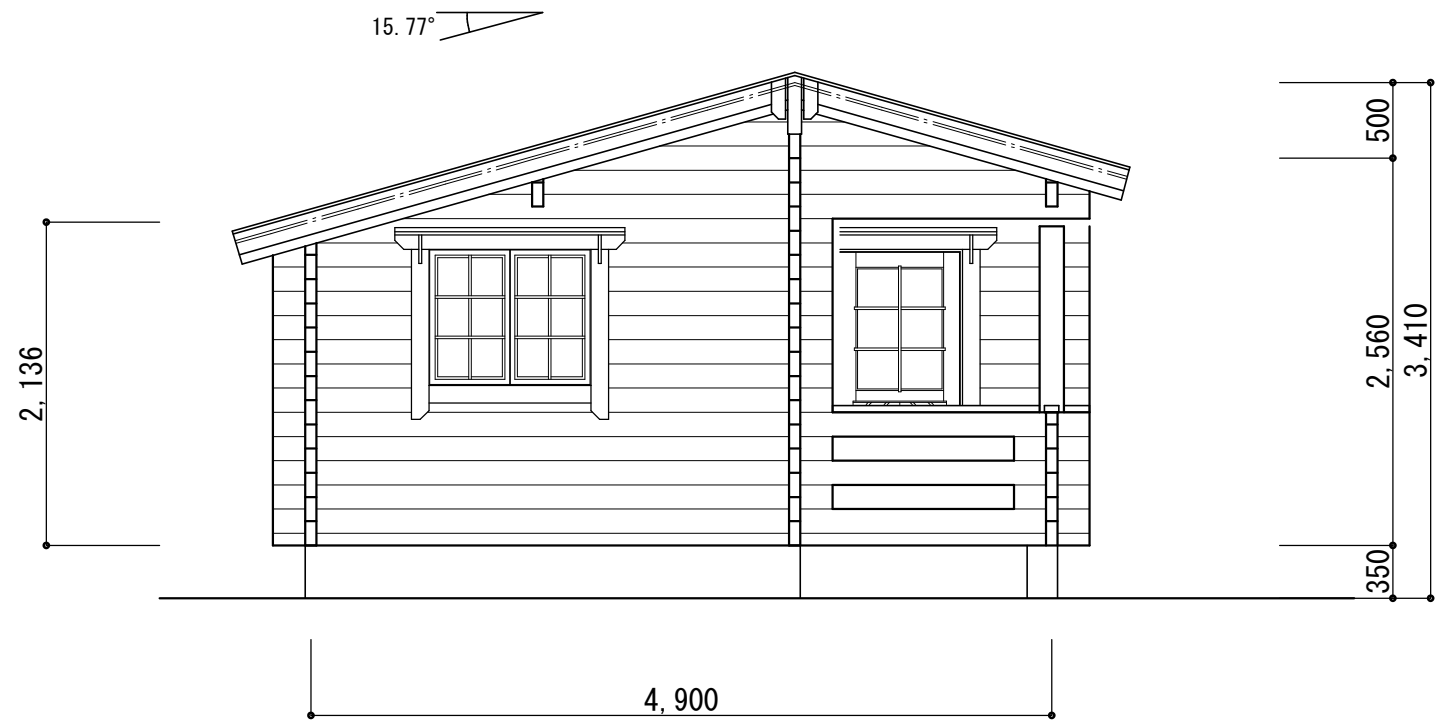
立面图 S=1/50
