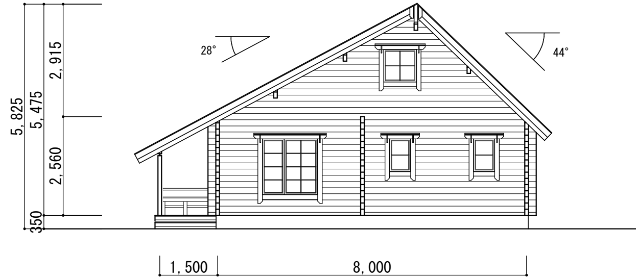
立面图 S=1/100
