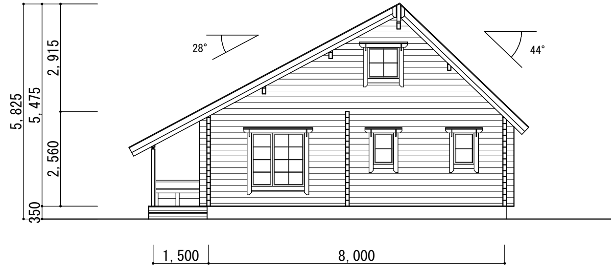
立面图 S=1/100
