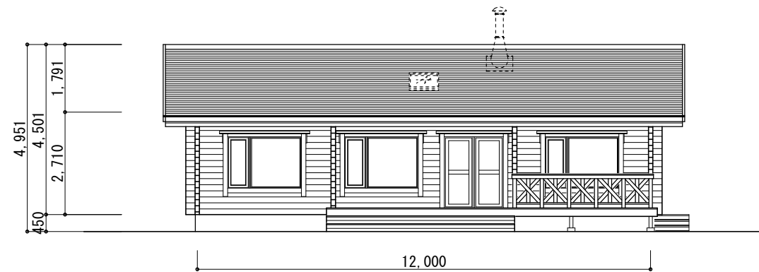
南側立面图 S=1/100
