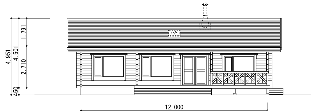
南側立面图 S=1/100
