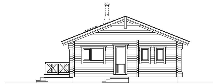
東側立面图 S=1/100
