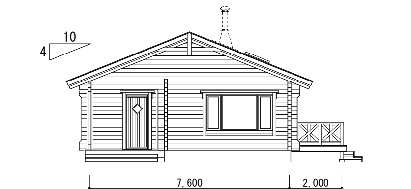
西側立面图 S=1/100
