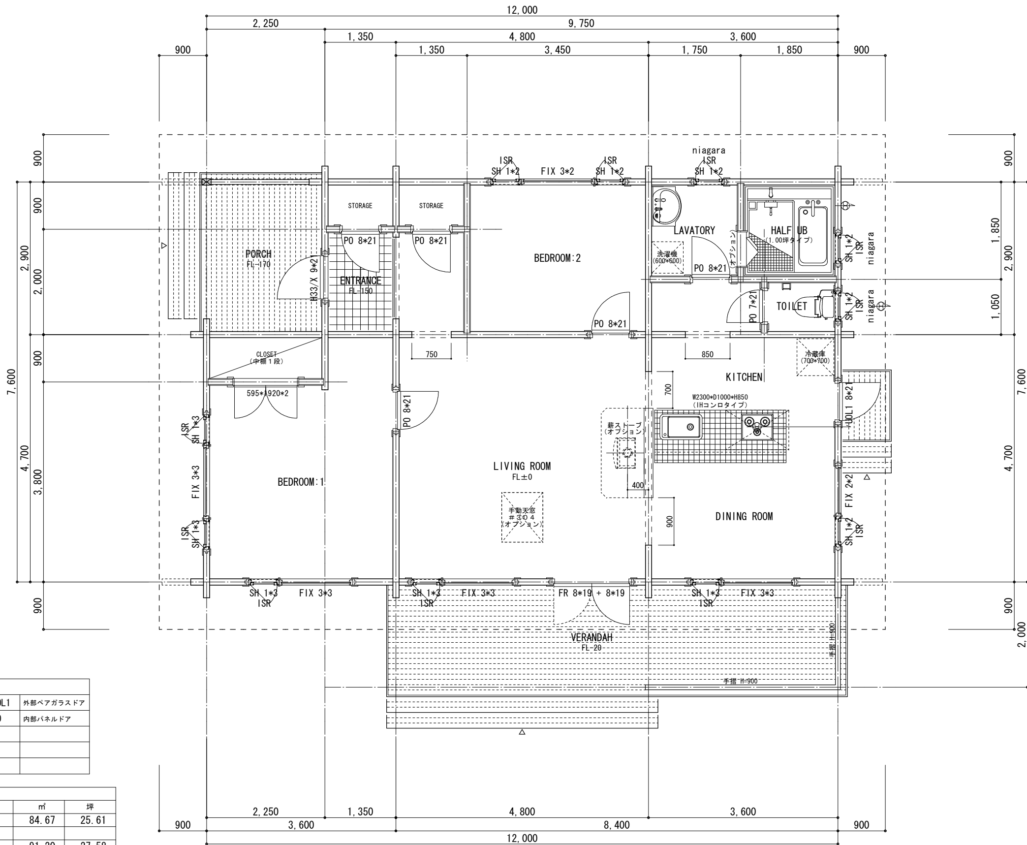
1階平面図 S=1/50
