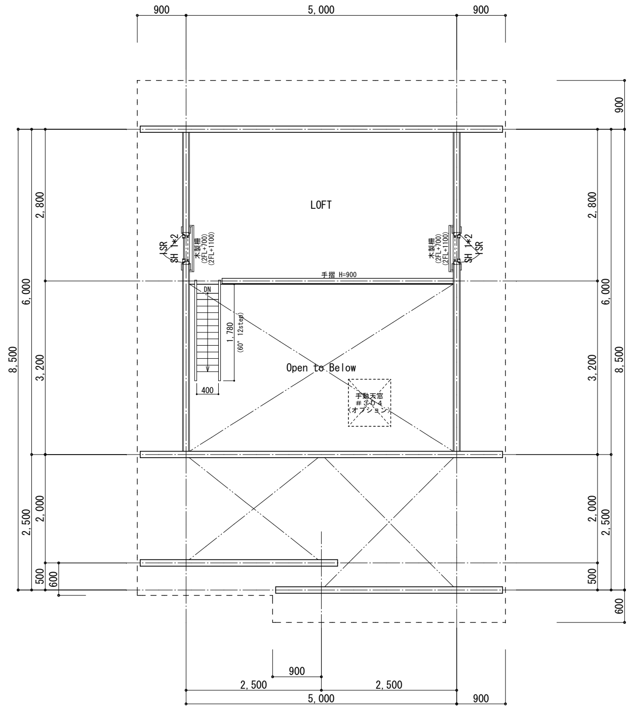
2階平面図 S=1/50
