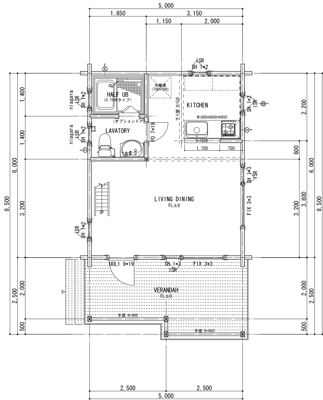
1階平面図 S=1/50
